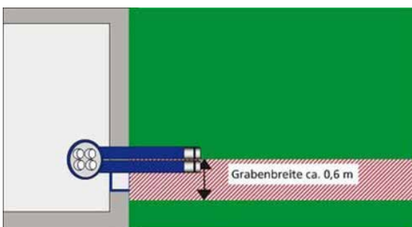
Gebäudeaußenseite
