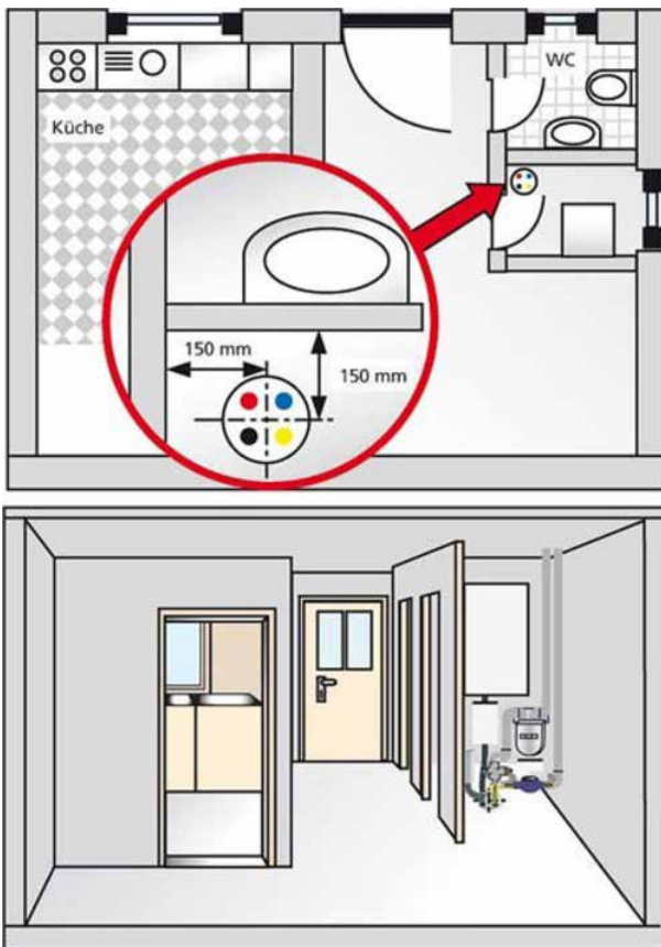
Gebäudeinnenseite
